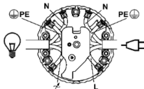
Anschluss-Skizze
