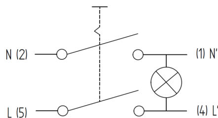
Anschlussbelegung, 2-polig, beleuchtet
